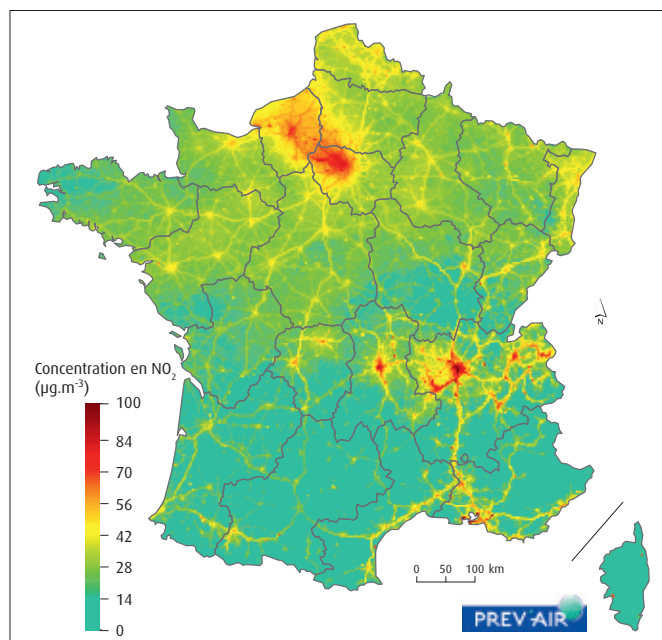
Carte 24 : concentrations moyennes journalières en NO 2 le 11 décembre 2013
