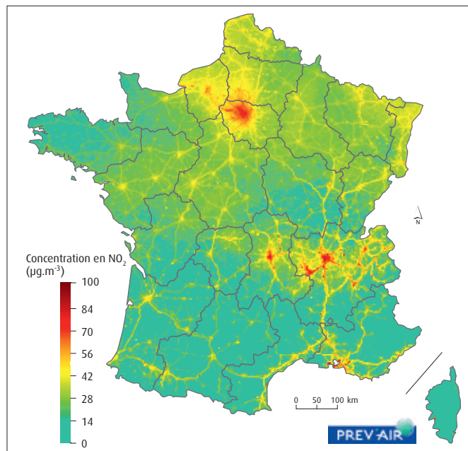
Carte 25 : concentrations moyennes journalières en NO 2 le 12 décembre 2013
