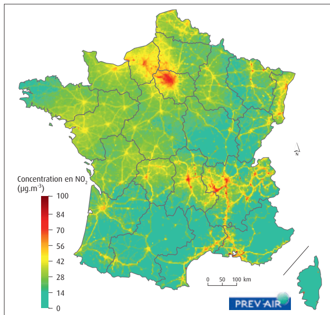
Carte 23 : concentrations moyennes journalières en NO 2 le 10 décembre 2013
