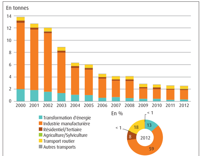
Graphique 19 : évolution des émissions françaises de Cd
