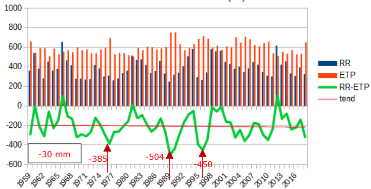
Précipitations (RR) et évapotranspiration (ETP) - avril à octobre Forêt de La Guerche (35)
